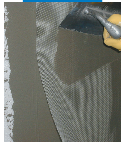
Εξομάλυνση θερμομονωτικών πλακών ενισχυμένων με υαλόπλεγμα που έχει ενσωματωθεί στη στρώση του Mapetherm AR1
